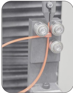
삽입 검사
